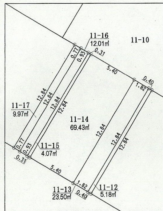
縮尺=1/250
