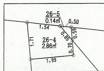
縮尺=1/100
