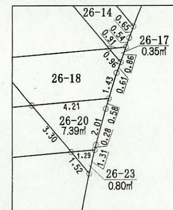
尺度=1/200
