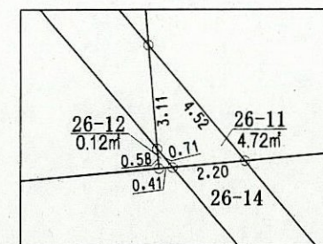
尺度=1/200
