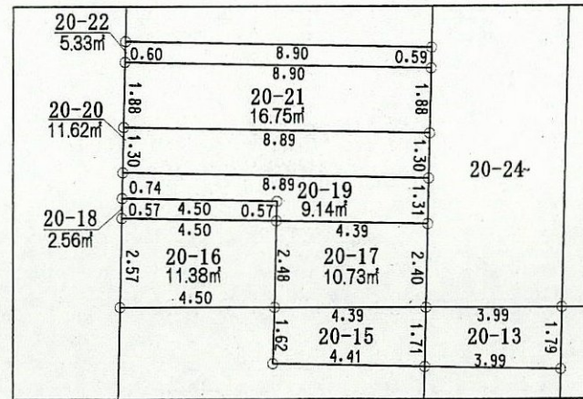
縮尺=1/200
