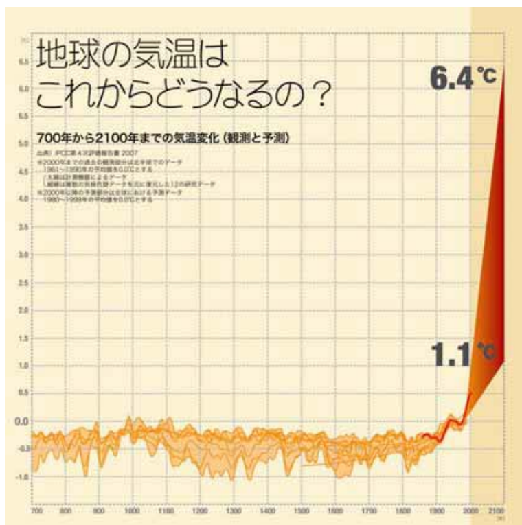
図6 地球の気温変化
