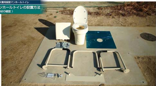
マンホールトイレ設置に必要な部材
