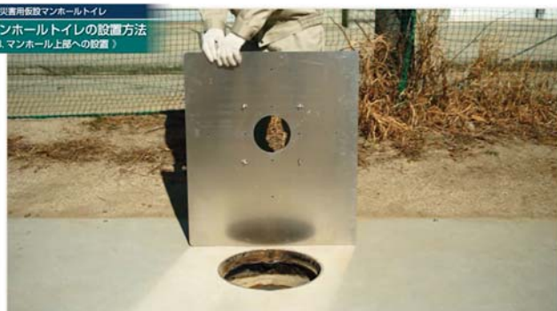
蓋を開けたマンホール上部にネジが突出した方を下にして床板を敷く
