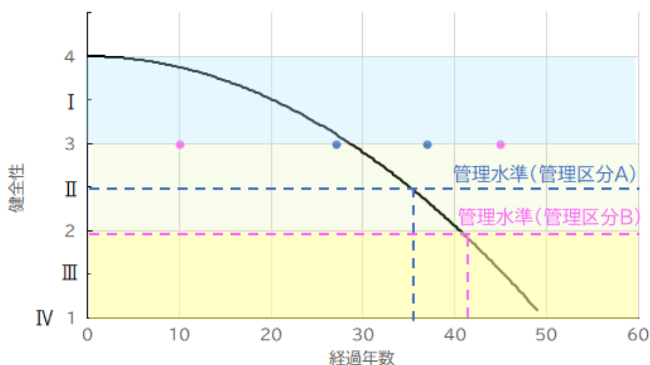
図 6-2 劣化曲線
