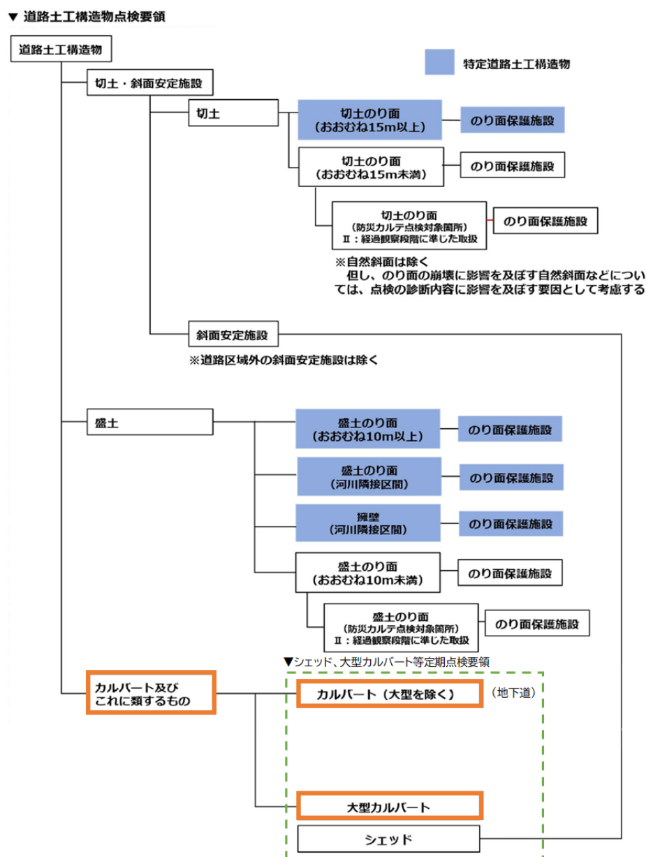
図 3-7 道路土工構造物の分類と適用範囲
