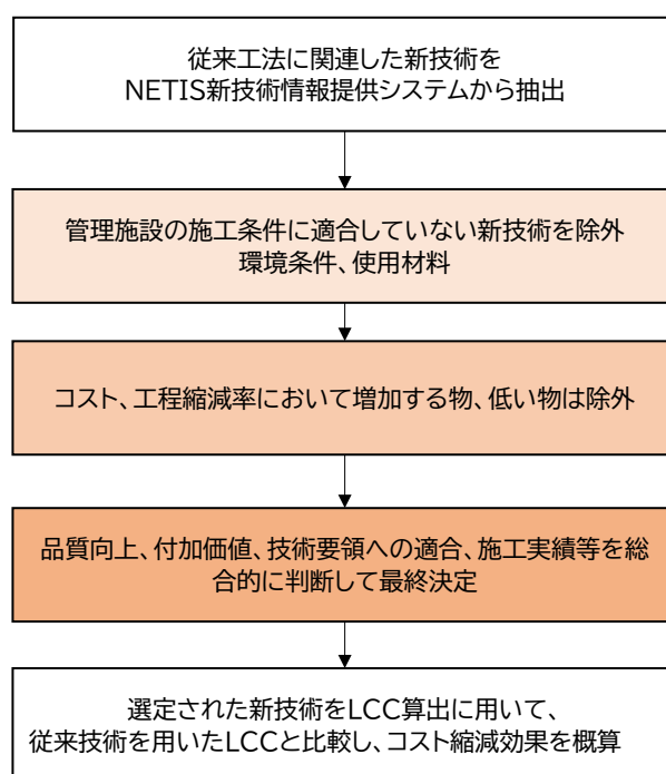
図 10-1 新技術(修繕)の選定フロー
