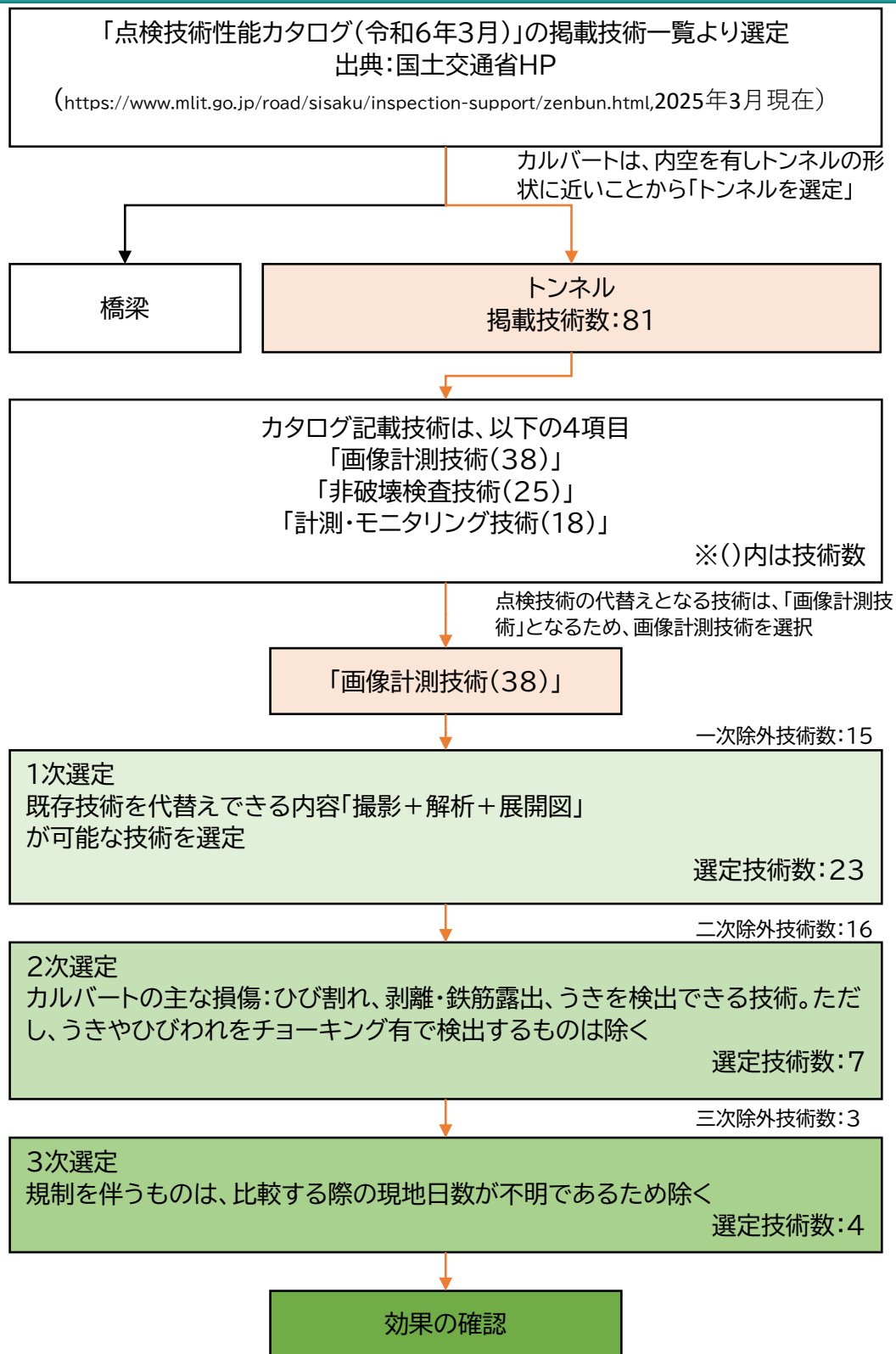
図 10-2 新技術(点検)の検討フロー
