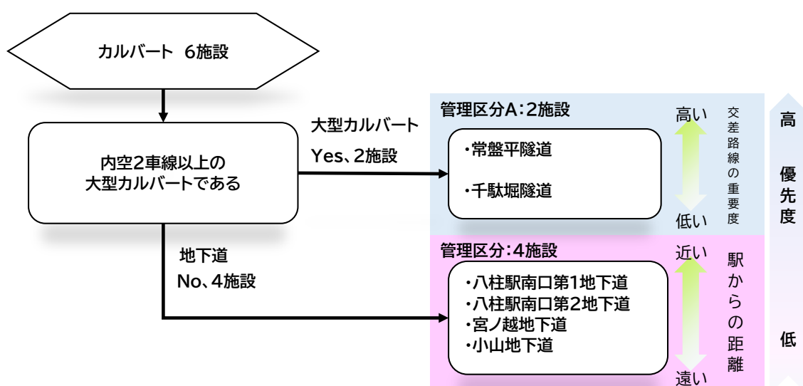
図 4-1 カルバートの維持管理区分の分類のフロー
