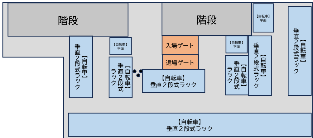
2階 平面図
