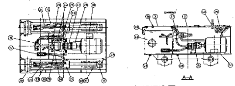
油圧バケット内部構造図
