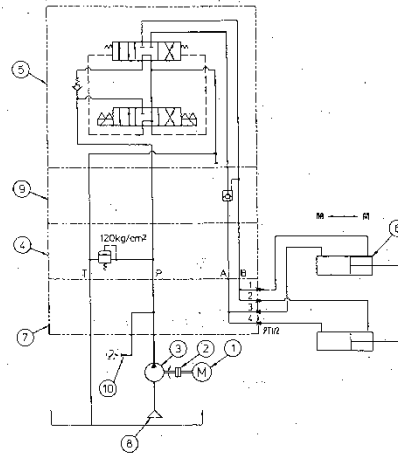
油圧図説明
