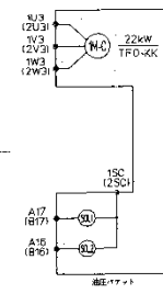
油圧バケット内電装回路図
