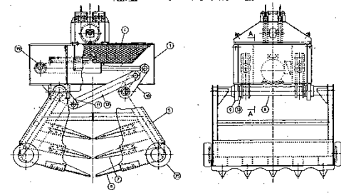
油圧バケット内部構造図
