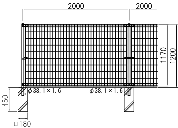
転落防止柵（プレキャストコンクリート）S=1/20 歩車道境界ブロック（180/205×250×600）S=1/5
