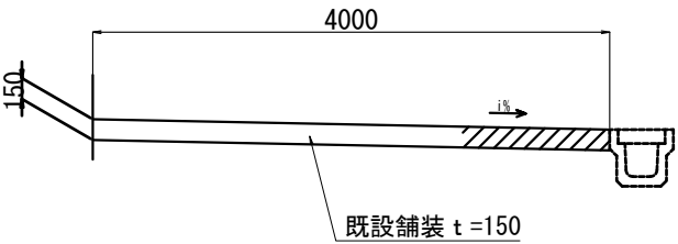
現況横断面図 (No. 5+15.5～No. 10)
