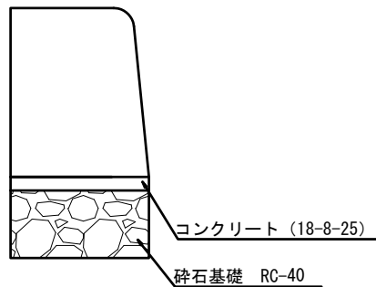
転落防止柵（プレキャストコンクリート）S=1/20 歩車道境界ブロック（180/205×250×600）S=1/5
