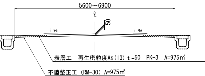
標準横断図 S=1/30
