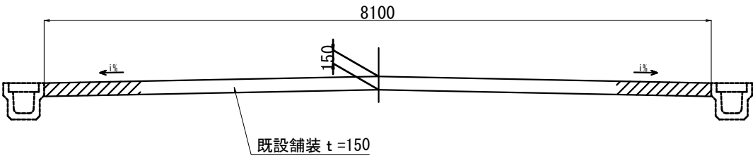
現況横断面図 (No. 0～No. 5+15.5、No. 10～No. 10+14.0)
