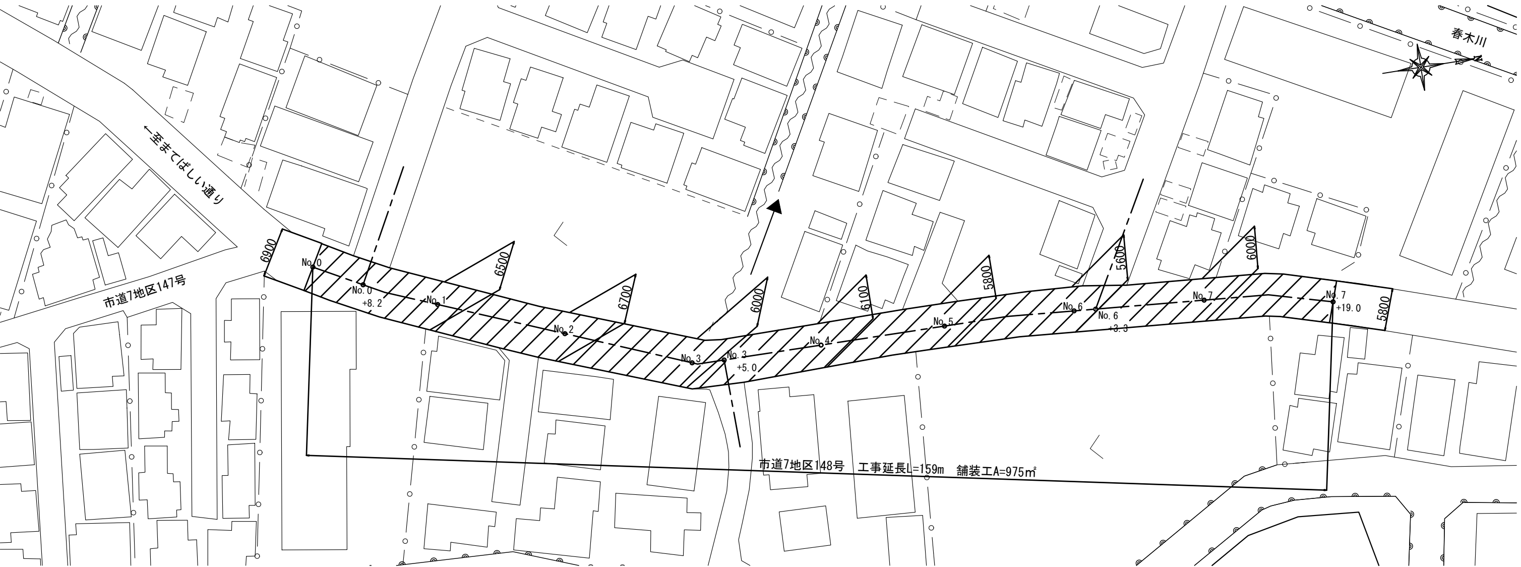
平面図 S=1/300
