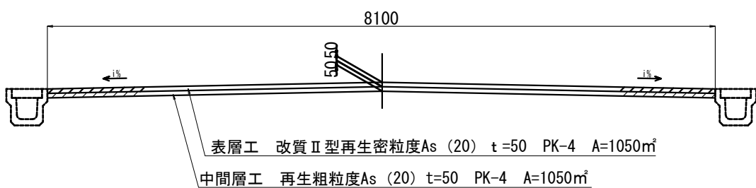
計画横断面図 (No. 0～No. 5+15.5、No. 10～No. 10+14.0)
