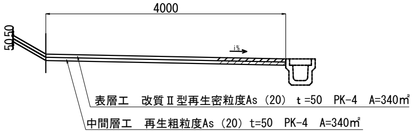
計画横断面図 (No. 5+15.5～No. 10)
