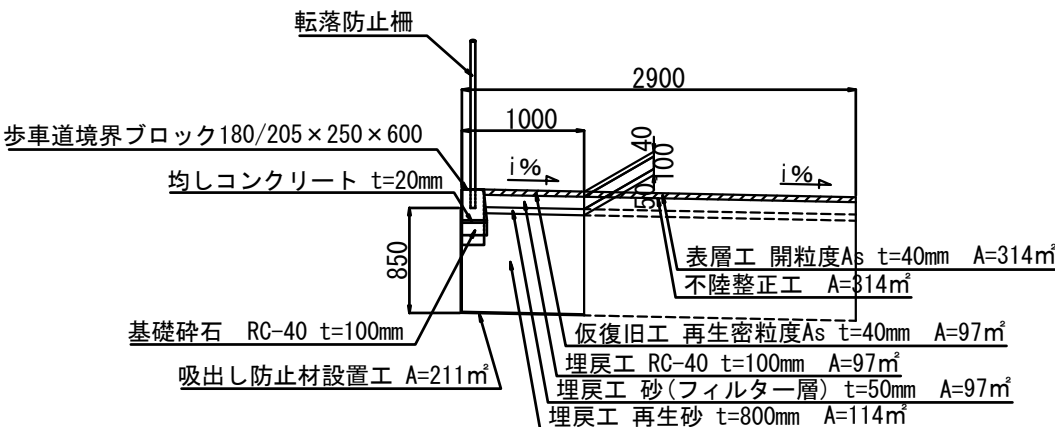
計画横断図
