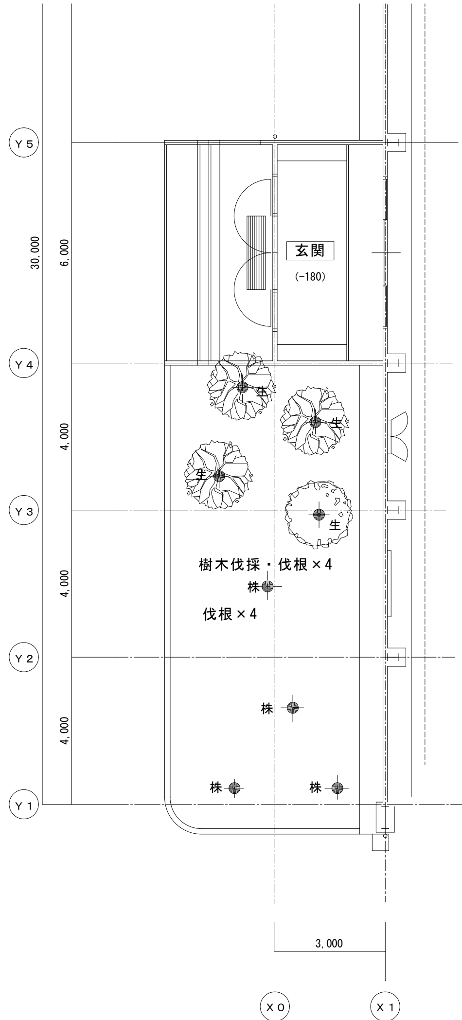
機器設置現状図
