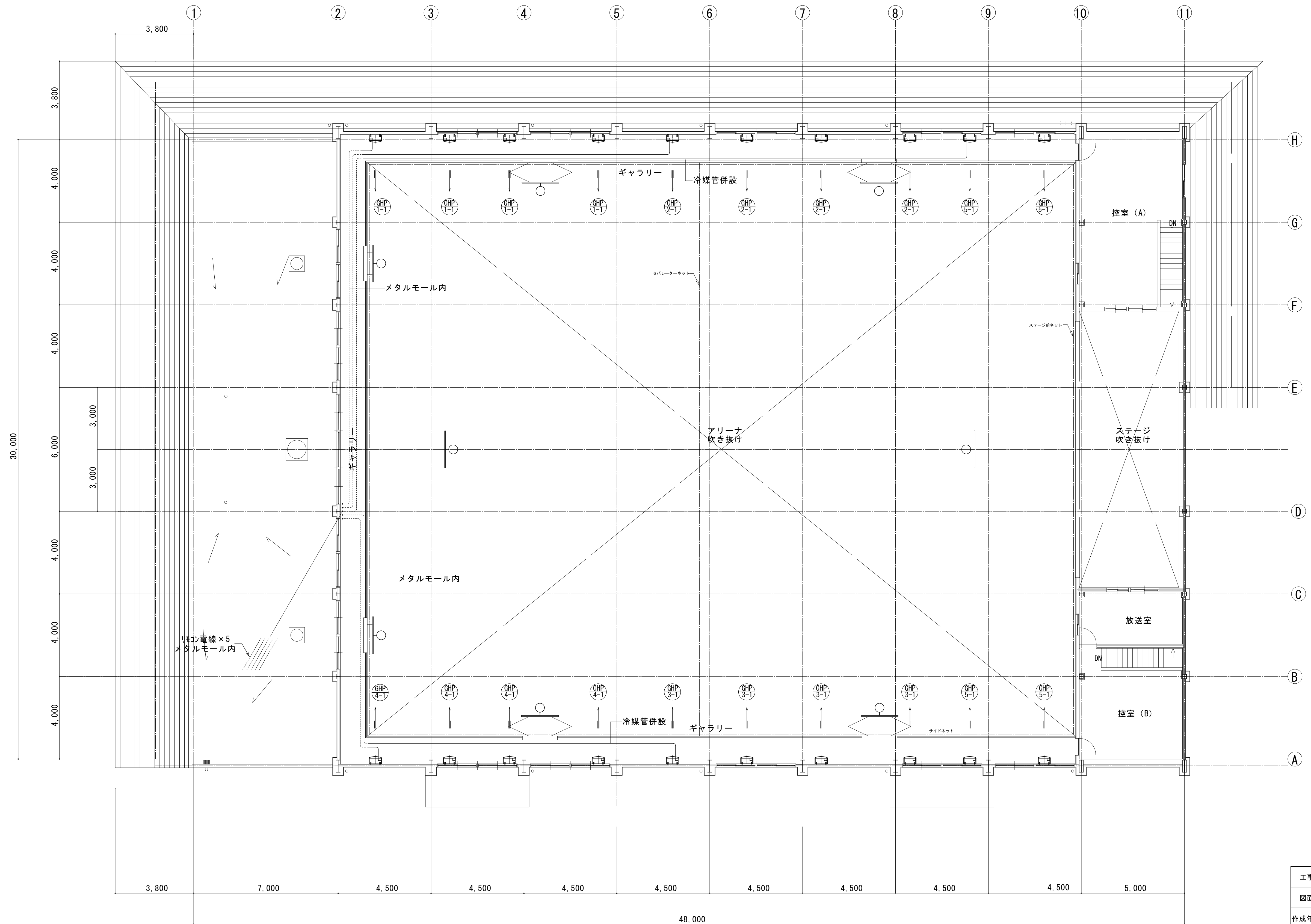
2階平面図 1:100
