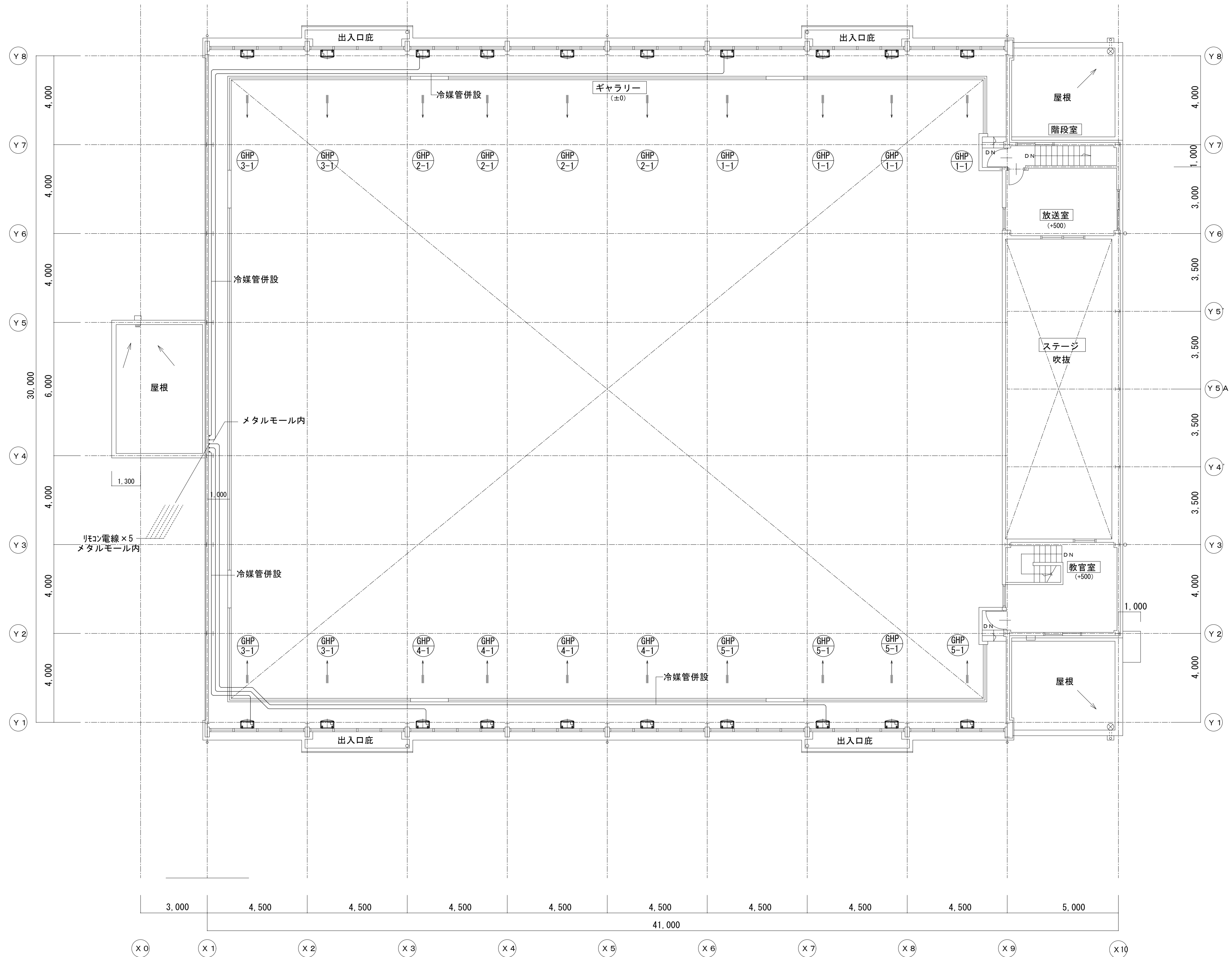
2階平面図 1:100
