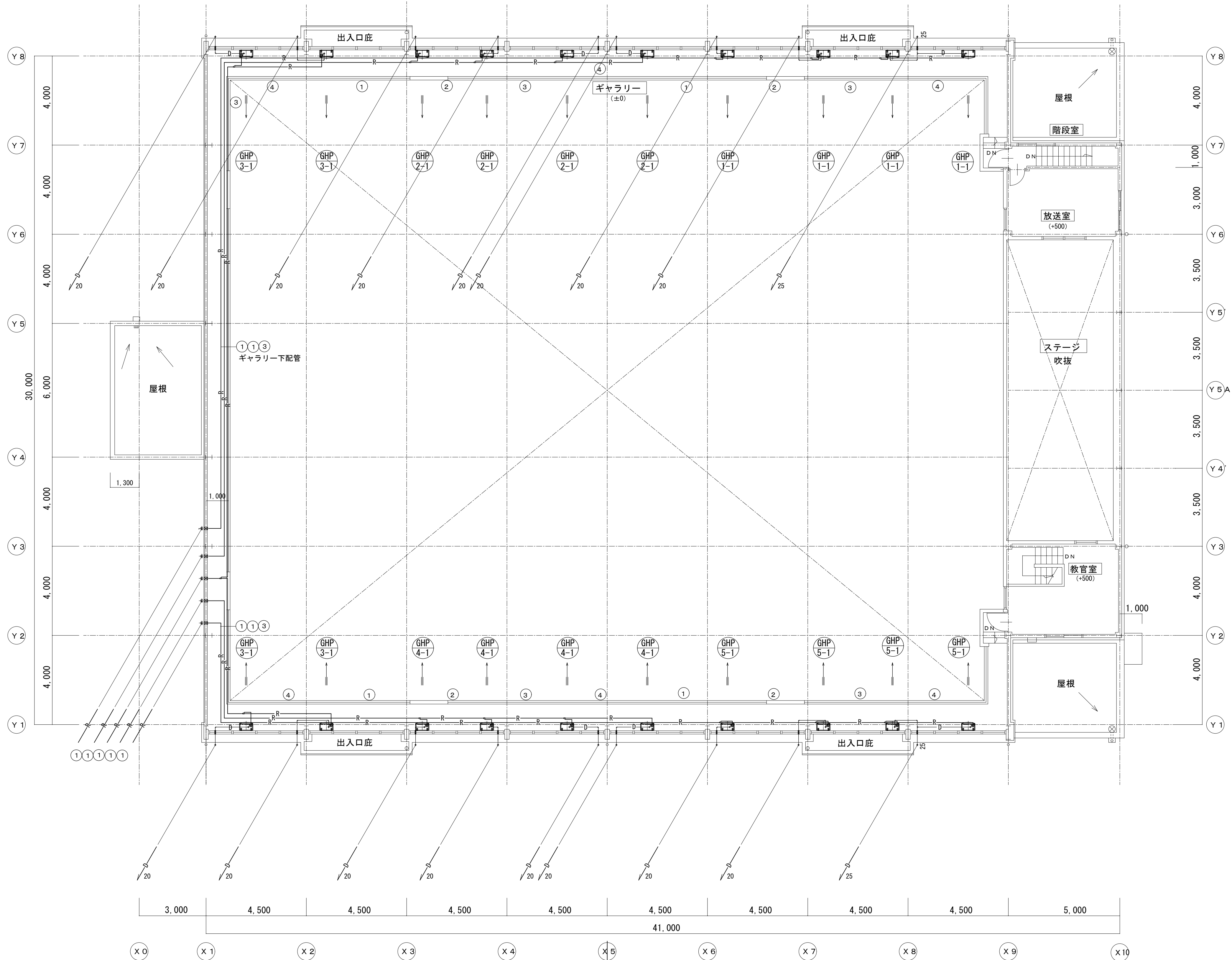
2階平面図 1:100
