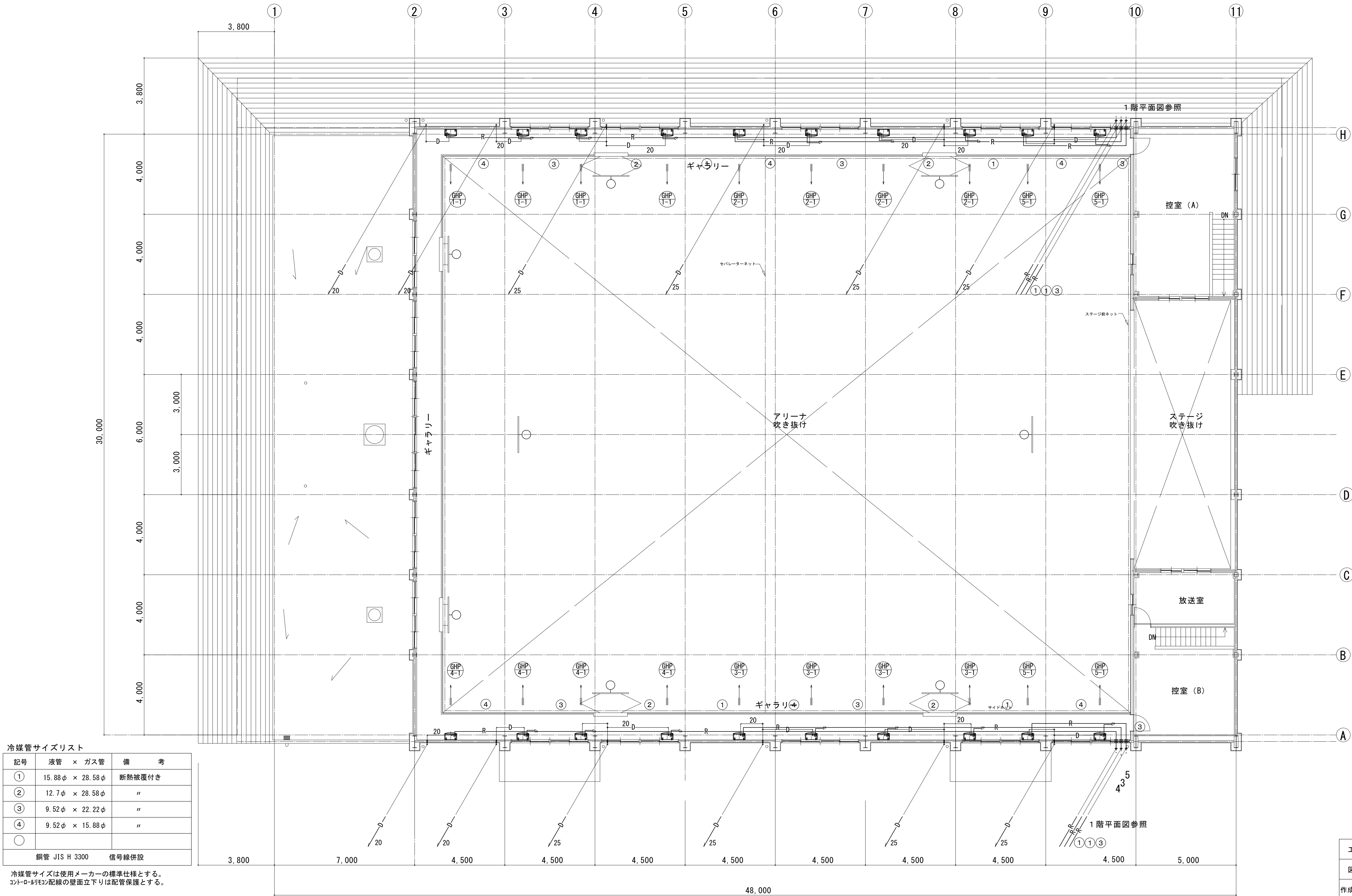
2階平面図 1:100
