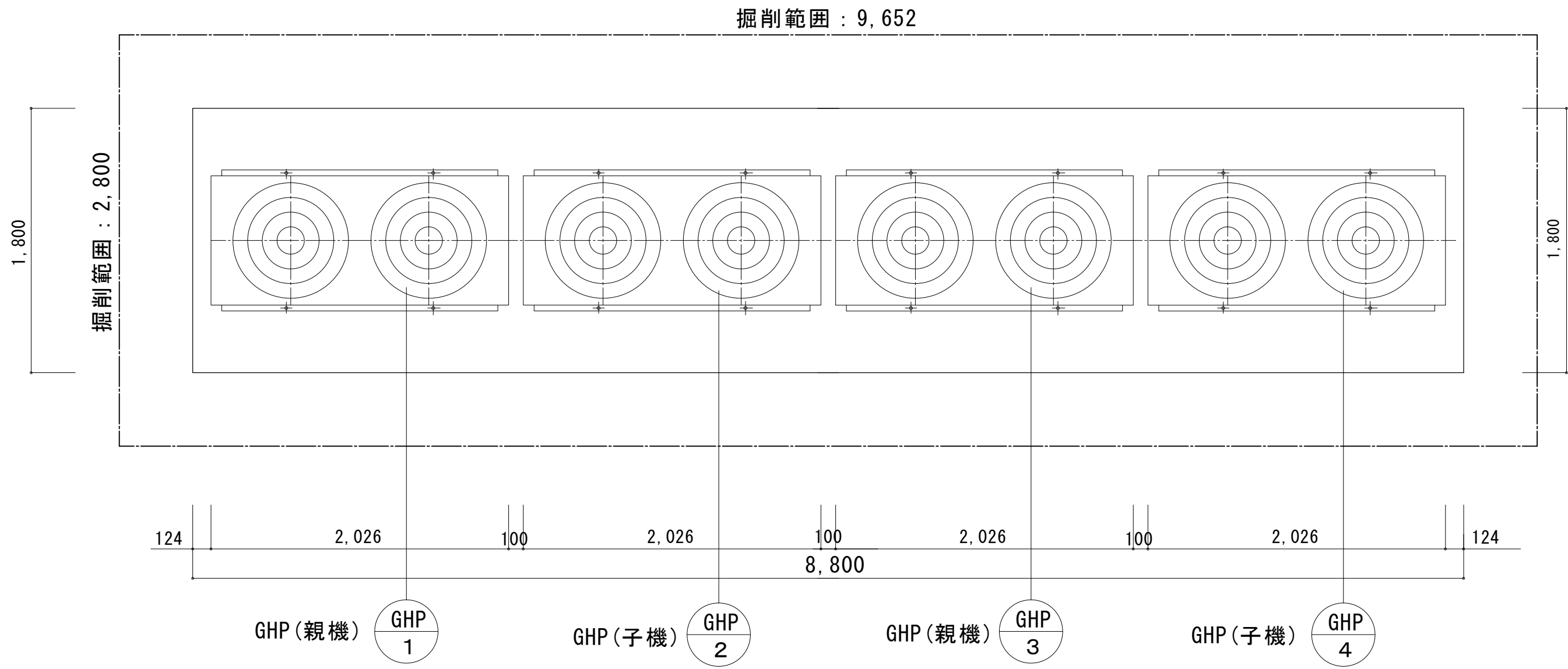
基礎タイプ E
