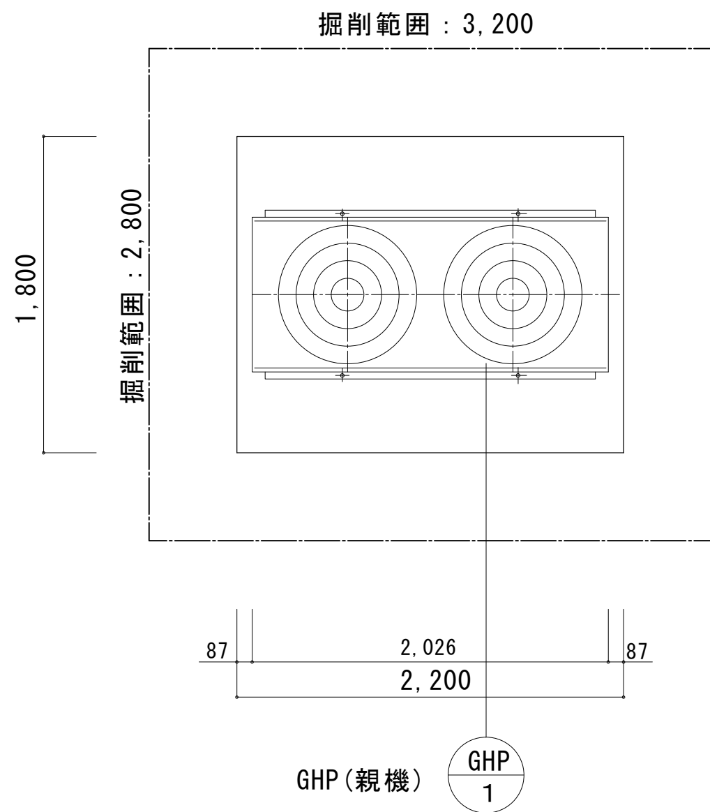
基礎タイプ C
