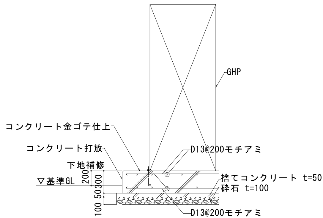
室外機基礎 標準配筋図 S=1:30
