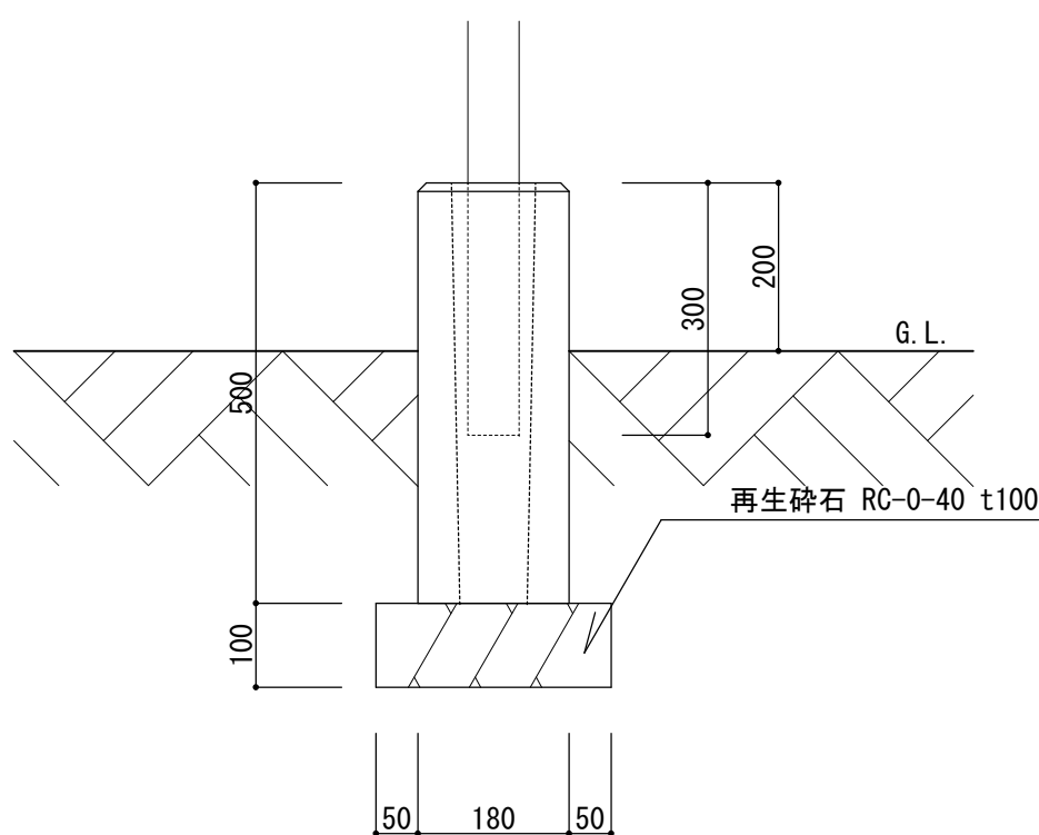
フェンス支柱基礎断面図 1:10
